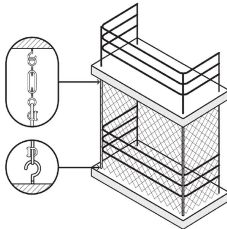
DETALLE DE HERRAJE DE TENSIÓN
